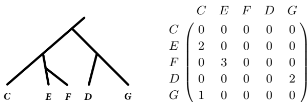
図 9: タイムスパン木の例とその行列表現
