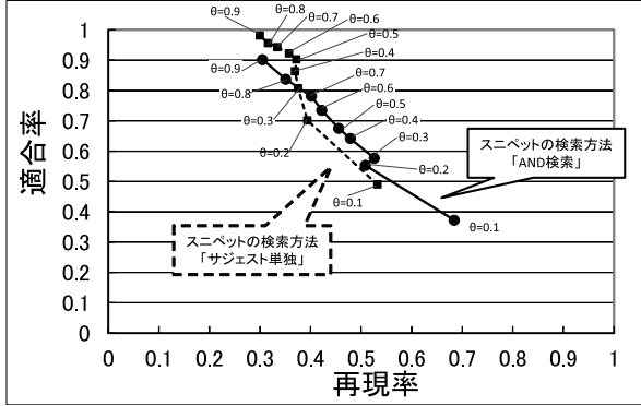
図 2: ウェブ検索者の情報要求観点の集約: 評価結果 (全検索対象分のマクロ平均)
