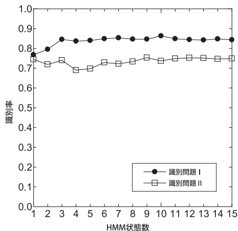
図 5 HMM 状態数-識別率グラフ
