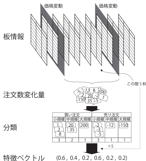
図 3 特徴抽出
