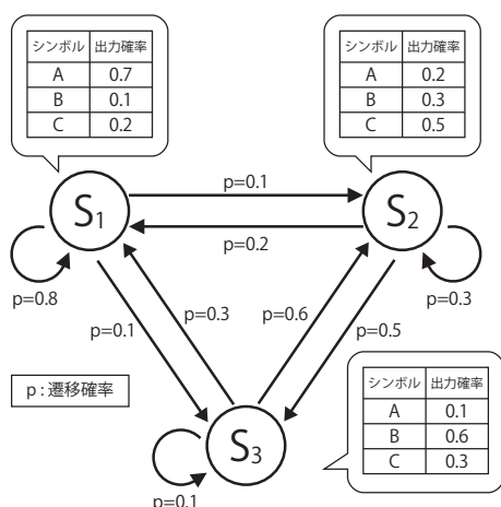
図 4 HMM
