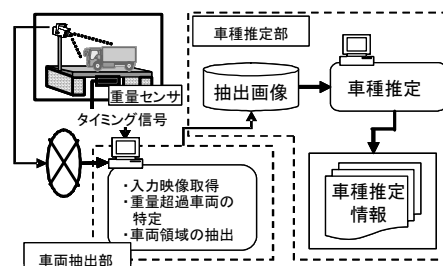
図3 重量超過車両検知システムの概要
