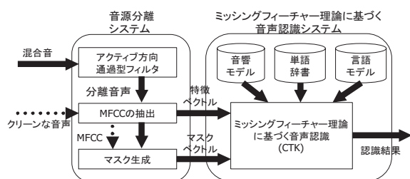
図 1: 複数同時発話認識を行うロボット聴覚システム
