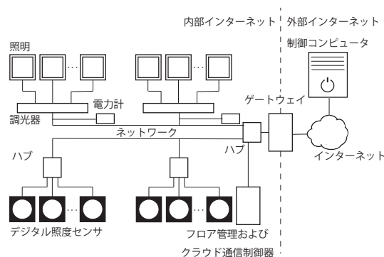
図 1: クラウド型知的照明システムの構成図
