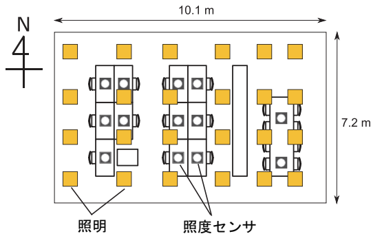
図 2: エコツェリアの照明と照度センサの配置図
