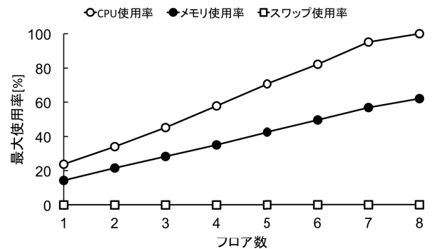
図 3: 負荷削減手法における制御コンピュータの負荷
