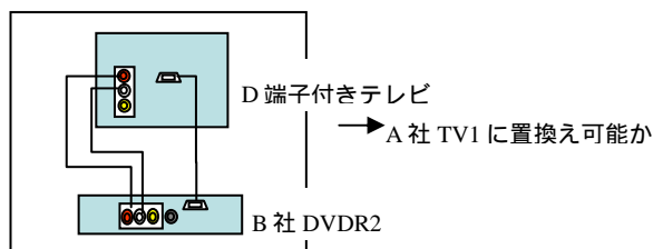
図5: D 端子付きテレビとの接続事例
